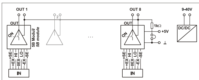
Funktionsschaltbild
